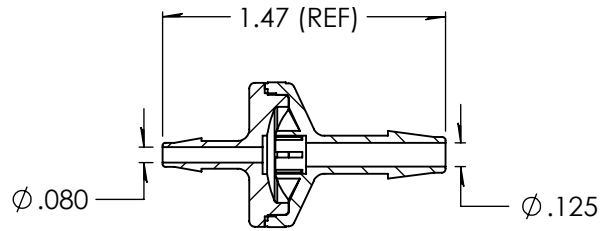
SECTION A-A
